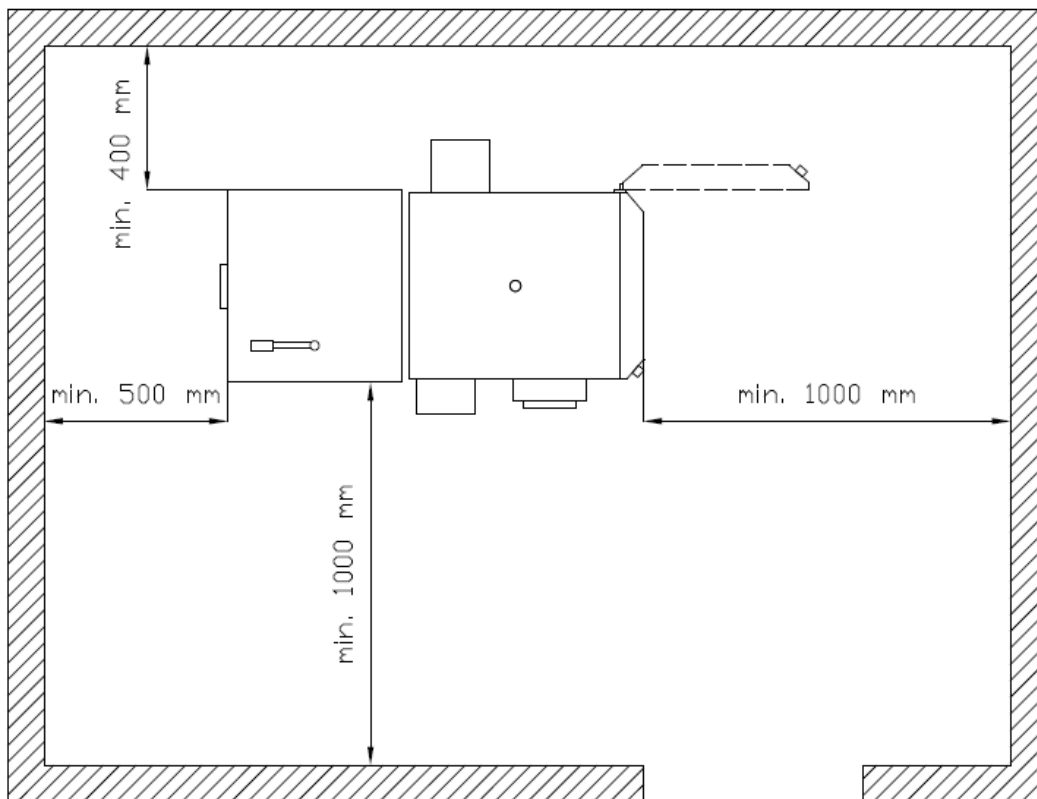
Příklad umístění kotle
